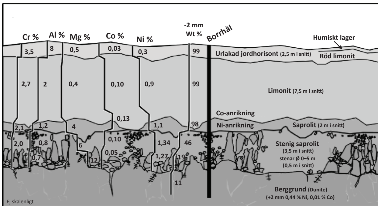
Figur 9. Profil genom en lateritmalmslag med kobolt i Ramufyndigheten, Papua Nya Guinea. Lateritprofilens huvudsakliga lager är illustrerade med minskande grad av vittring ned till det underliggande berget. Illustrationen visar hur metallhalter varierar i den extremt vittrade jordprofilen och var kobolthalterna är högst. Källa: Modifierad från Queen m.fl. (2001).
