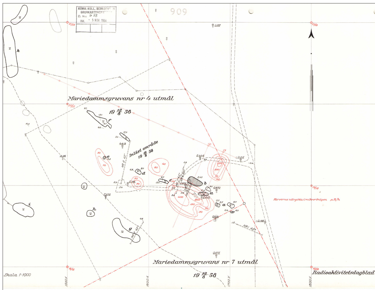
Figur 16. Radioaktivitetsdagblad över Mariedamms gruvor upprättad 1964 efter avslutade mätningar 1958. Radioaktivitetsmätningar ( \mu\text{R}/\text{h} ) visar förhöjd strålning inom röda områden. På många håll har uranförande järnmalm påträffats och bland några gamla kända gruvområden kan nämnas till exempel Persbergs Odalfält (Filipstads kommun) och Bispsbergsfältet (Säters kommun).
