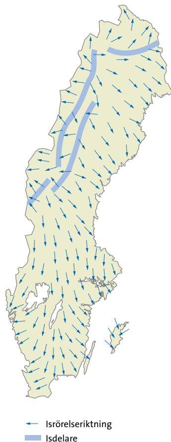
Figur 4. Genom att känna till den senaste inlandsisens rörelseriktning kan man spåra varifrån intressanta block kommer.
