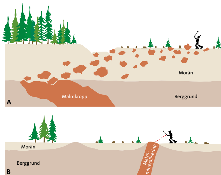
Figur 6. Blockletning ger stora chanser att hitta hittills oupptäckta, jordtäckta malm- och industrimineralförekomster. Som figur A visar kan block i ytan "skvallra" om en malkropp längre ned under jordlagren.
