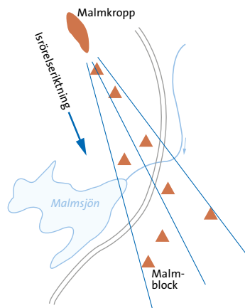
Figur 5. Inlandsisen tog ofta med sig flera block, som har lämnats kvar i form av en blocksvans. Ju tätare blocken ligger, ju närmare ursprungsplatsen är man.
