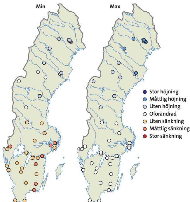
Figur 15. Skillnad mellan högsta och lägsta grundvattennivåskillnad för morän under våren för utsläppsscenario RCP 8.5, perioden 2069–2098. I södra och mellersta delen av landet är det stor skillnad mellan lägsta (till vänster) och högsta (till höger) beräknad nivåskillnad i förhållande till referensperioden.
