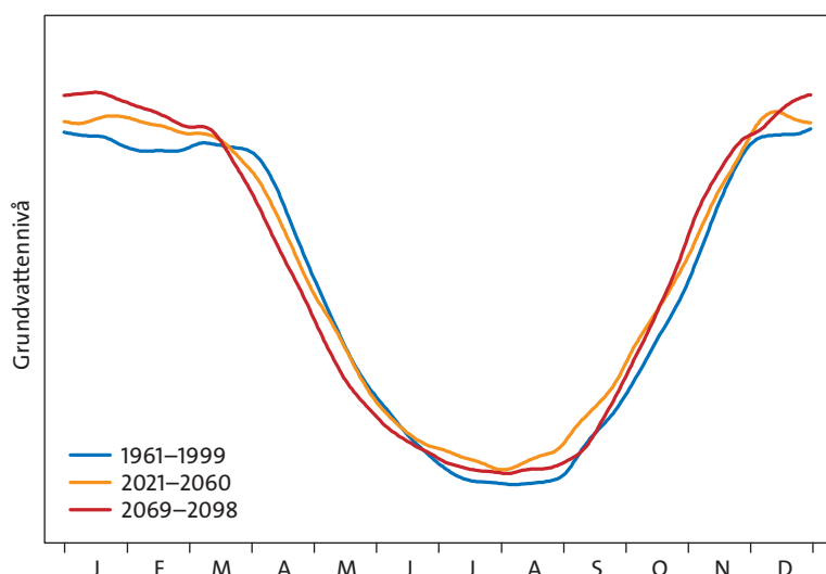
Figur 19. Dygnsmedelvärden för station (52_13) på västkusten, södra Sverige, i snabbreagerande magasin. Diagrammet visar perioderna 1961–1999, 2021–2050 och 2069–2098 för RCP 8.5.
