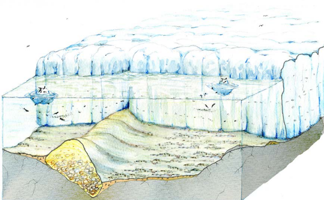
Figur 24. Rullstensåsarna avsattes av inlandsisens smältvatten i tunnlar under isen. På bilden syns hur inlandsisen drar sig tillbaka i ett område under högsta kustlinjen varvid en rullstensås bildas. Illustration: Art Anna.
