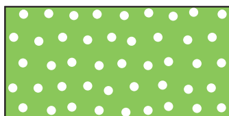
Figur 23. Isälvssediment symboliseras med en grön färg och på de mer detaljerade kartorna anges vilken kornstorlek som dominerar jordarten.
