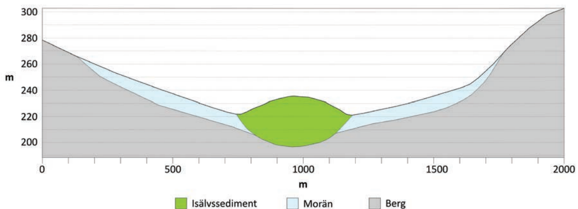
Figur 49. Profil 2 visar en dalgång med en isälvssavlagring belägen ovanför högsta kustlinjen.
