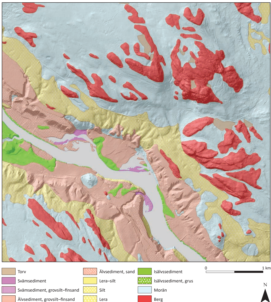
Figur 11. Jordarternas fördelning i en norrländsk dalgång under den högsta kustlinjen. Höjdområdena domineras av hållmark och morän. Dalgången domineras av olika typer av vattenavsatta sediment. I dalgångens mitt finns ett vattendrag som delvis eroderat tidigare avsatta sediment. I kartan syns även en skuggning från Lantmäteriets höjdmödel. I denna skuggning syns även diken, vägar med mera vilka är en effekt av olika mänskliga aktiviteter.
