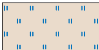
Figur 41. På detaljerade jordartskartor redovisas områden där gyttja förekommer. På de mer översiktliga kartorna symboliseras gyttja på samma sätt som torv.
