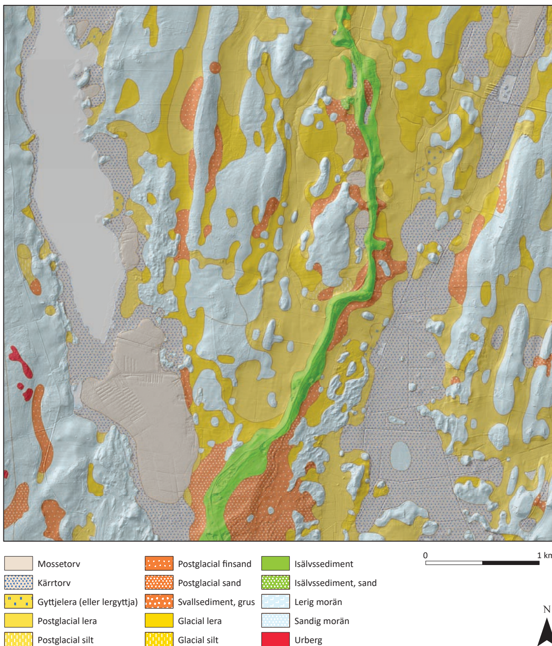
Figur 12. Jordarternas fördelning i ett område beläget under högsta kustlinjen i Mellansverige. Området är relativt flackt men de lite högre områdena domineras av morän samt en markant rullstensås. Lägre delar av terrängen domineras av olika typer av lera samt torv. Kring åsen finns sandavlagringar som avsatts då åsen bearbetades av vågor i samband med landhöjningen. I kartan syns även en skuggning från Lantmäteriets höjdmodell. I denna skuggning syns även diken, vägar med mera vilka är en effekt av olika mänskliga aktiviteter.
