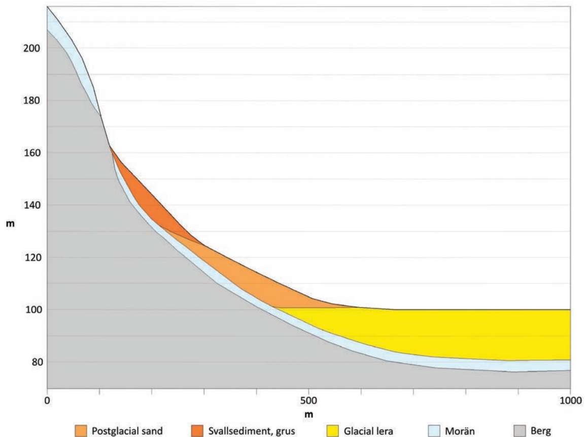
Figur 51. Profil 4 visar en sluttning som delvis ligger ovanför högsta kustlinjen (HK). Vid HK har jordtäcket eroderat bort och blottlagt berget. Det eroderade materialet har omlagrats och utgöt sand- och grusavlagringar i sluttningen nedanför HK.
