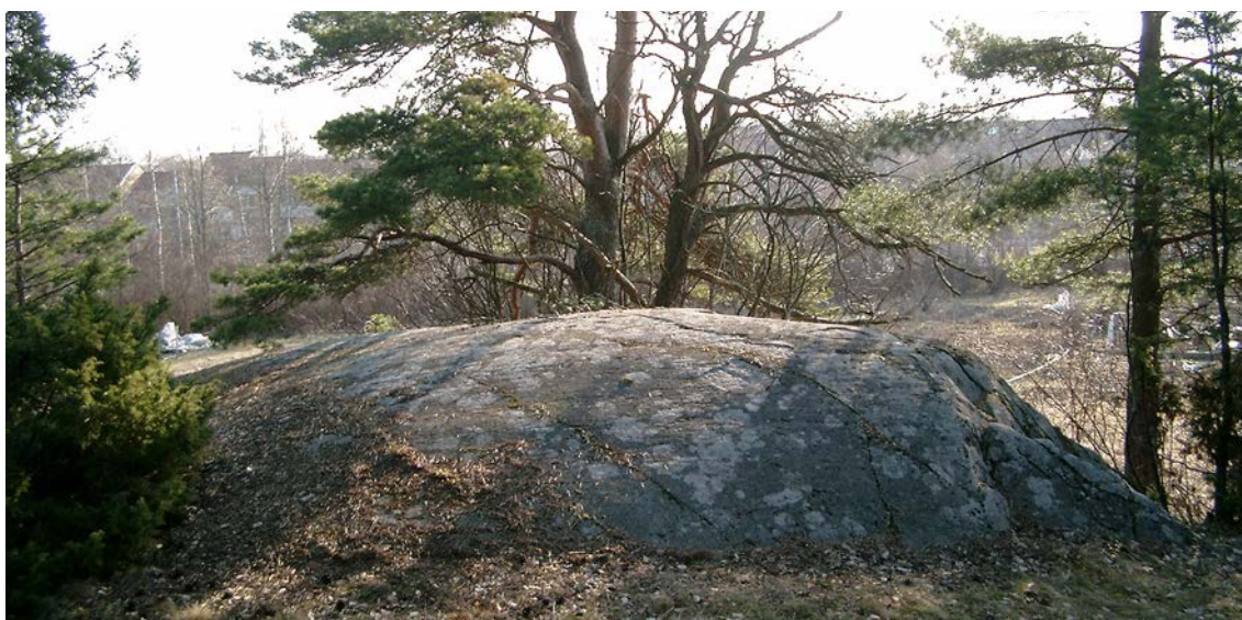
Figur 14. Rundhällar bildas som en följd av inlandsisarnas erosion av berggrunden. De har en relativt slät sida som vetter mot det håll som inlandsisen rört sig ifrån och en brantare sida som vetter åt andra hållet. Inlandsisen har rört sig över den släta sidan och material som varit infruset i isen har slipat ytan vilket gör att det ofta finns isräfflor på denna sida. Då isen rört sig över den brantare sidan har den frusit fast mot underlaget vilket lett till att material från berggrunden kunnat brytas loss och transporterats vidare av isen. Foto: Gustav Sohlenius.
