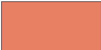
Figur 16. På jordartskartan symboliseras vittringsjord med denna färg.
