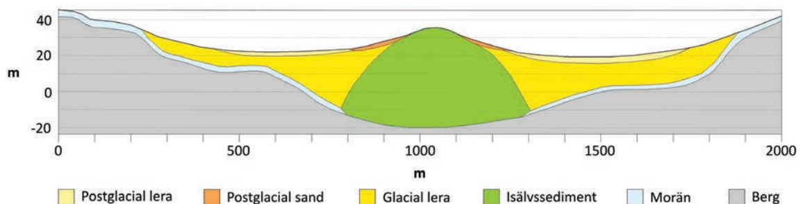
Figur 48. Profil 1 visar en genomskärning av en dalgång med en isälvssavlagring belägen under högsta kustlinjen.
