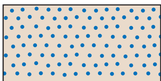
Figur 42. På detaljerade jordartskartor symboliseras mossetorv och kärrtorv på olika sätt. På de översiktliga kartorna används en gemensam symbol.
