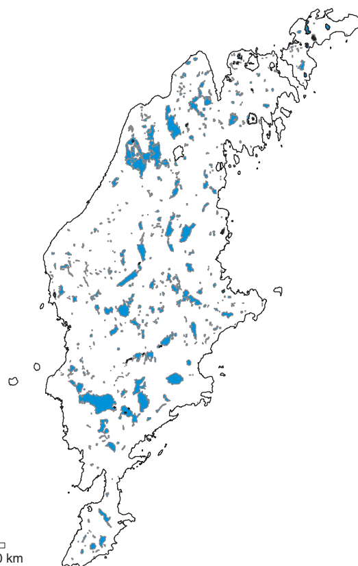
Figur 10. Uppskattad areal myrmark på 1700-talet. Underlag, skattningskarta från Länsstyrelsen Gotland. I stort sett samtliga områden är påverkade av dikning då de används som odlingsmark.
