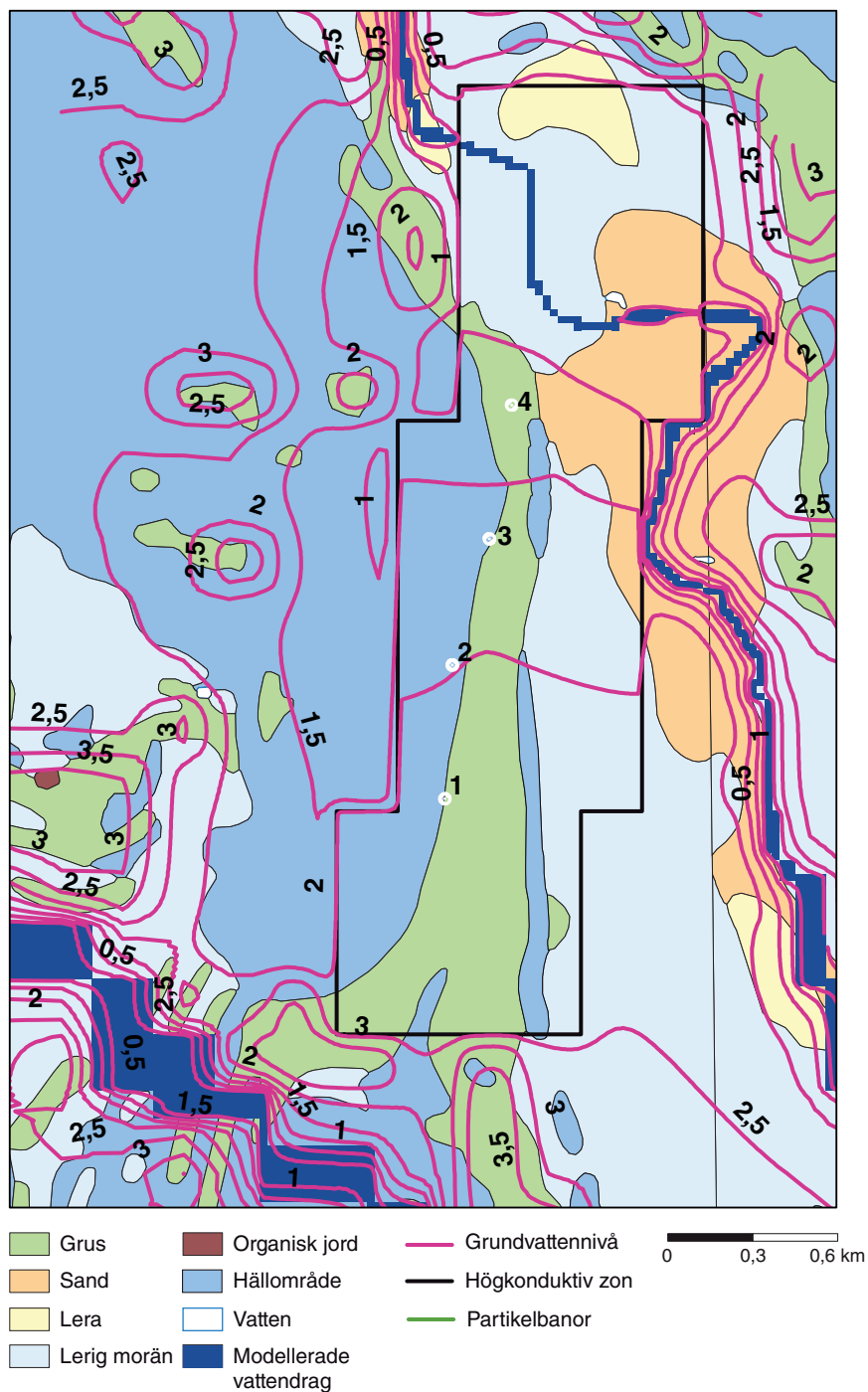
Figur 4. Grundvattenavsänkning jämfört med dagens situation efter 10 års drift av ett scenario med halvårsvis förstärkt infiltration (vinter) i utspridda dammar och halvårsvis ökat uttag (sommar). Grundvattenavsänkningen (lila ekvipotentiallinjer) påverkar ett större område runt infiltrationsbassängerna och brunnarna.
