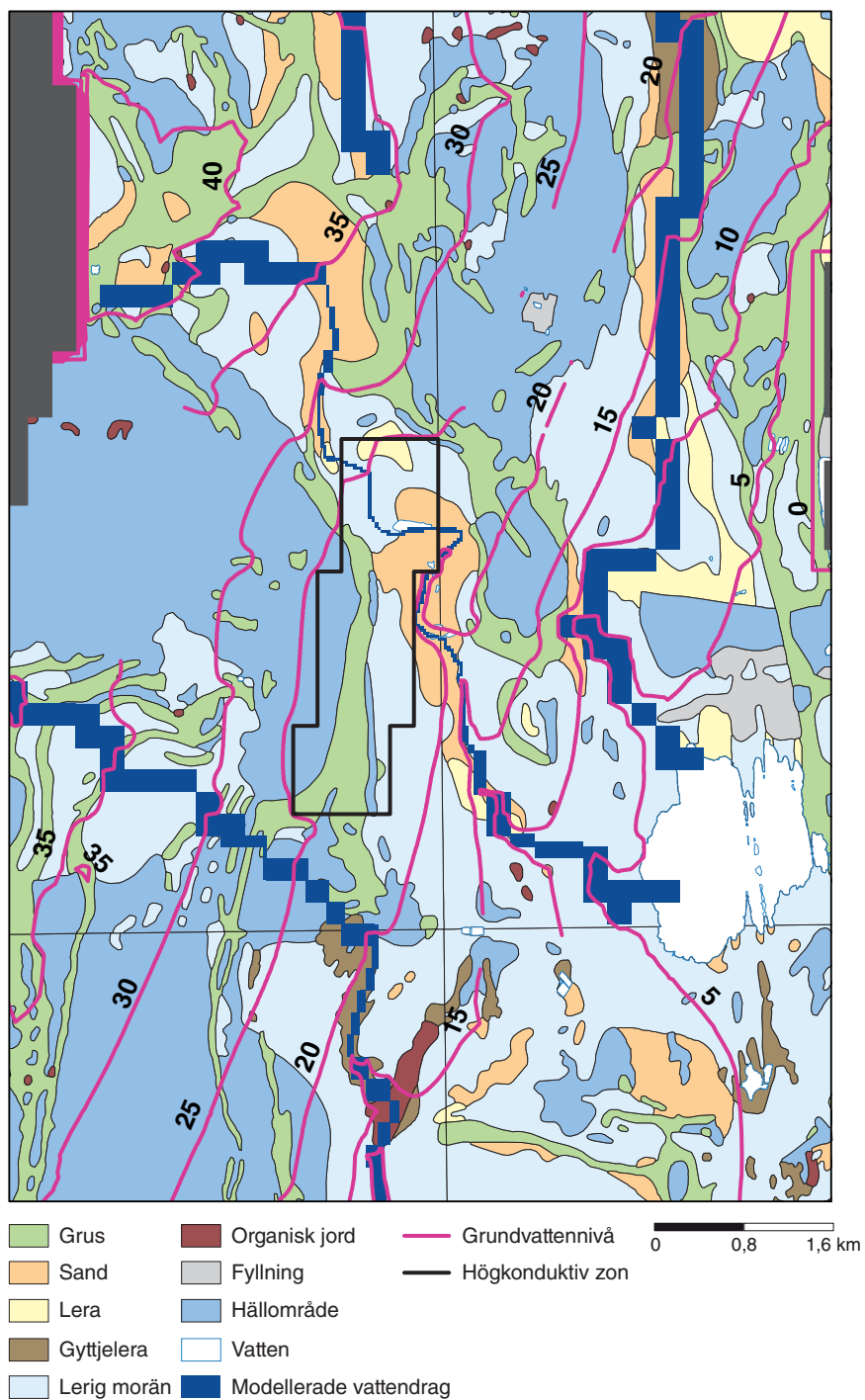
Figur 2. Grundvattennivåer (lila ekvipotentiallinjer) vid befintligt uttag. Naturlig grundvattenbildning. De vattenförande dikena (blå celler) som är belägna närmast uttagsbrunnarna och som ingick i vattenbalansredovisningen är mörkblå. Den högkonduktiva zonen markeras av grå linje.
