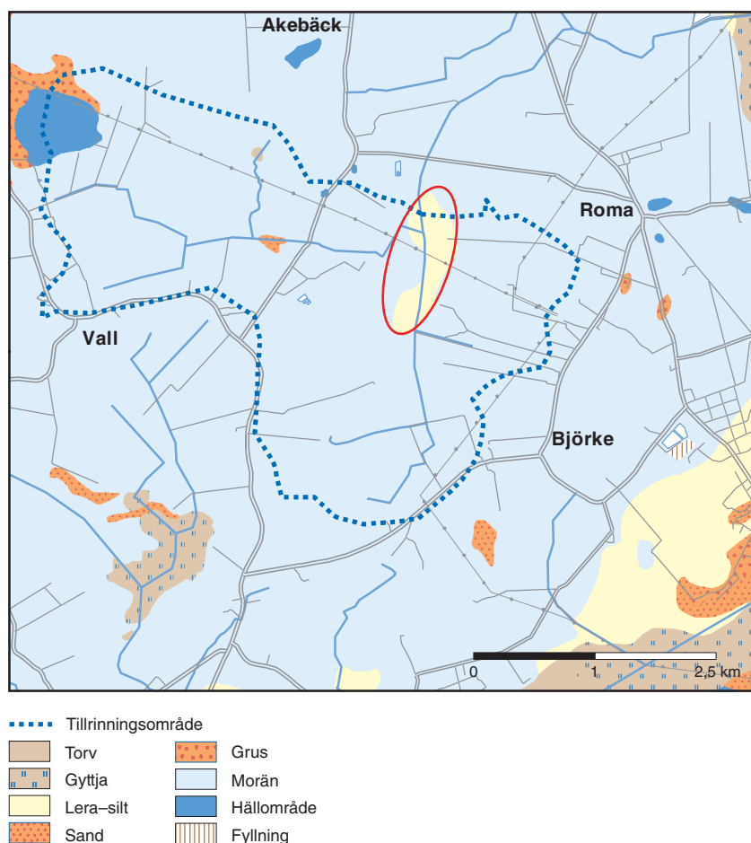
Figur 49. Figuren visar vattentächtsbrunnarna vid Roma. Uppskattat tillrinningsområde för det dike som rinner strax väster om Busarvebrunnarna, samt möjligt område för potentiell våtmarksanläggning (röd oval). Underlaget är SGUs jordartskarta.
