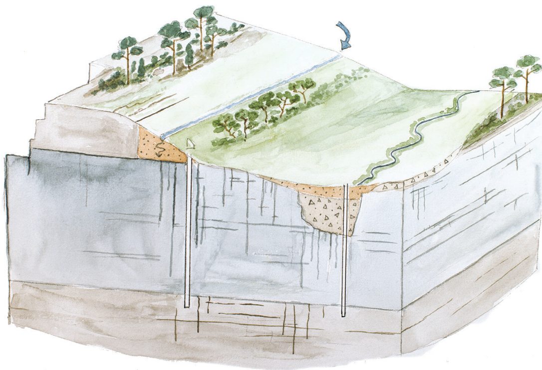
Figur 27. Principskiss på infiltrationsmöjligheter för förstärkt grundvattenbildning i anslutning till vattentäkten i Filehajdar. Notera att figuren är utdragen i höjddledd för att förtydliga de geologiska förhållandena.
