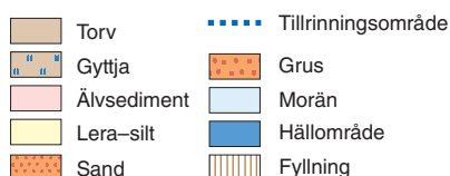
Figur 41. Jordartskarta över närområdet för vattentäkten i Kapellshamn. Den streckade linjen visar tillrinningsområdet för det dike som avvattnar vattentäkten närområde.
