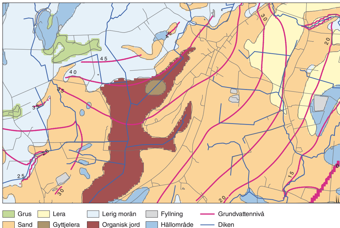
Figur 1. Grundvattennivåer (rosa ekvipotentiallinjer) vid befintligt uttag. Naturlig grundvattenbildning. Skala ca 1:20 000.
