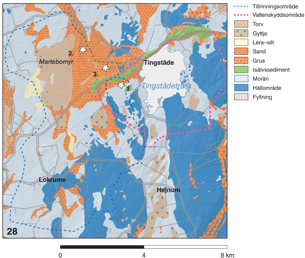
Figur 28. Jordartskarta över Tingstade träsk's närområde med höjddata i bakgrunden. Rosa streckad polygon motsvarar vattenskyddsområdets yttre gräns. Blå streckade linjer är tillrinningsområden som diskuteras i texten. De markerade stjärnorna är de områden lämpliga för infiltration som diskuteras i texten, punkterna symboliserar vattentäcksbrunnarna.
