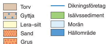
Figur 34. Jordartskarta över närområdet till vattentäkten i Lärbro. Röda ovaler markerar hypotetiska våtmarkslägen.
