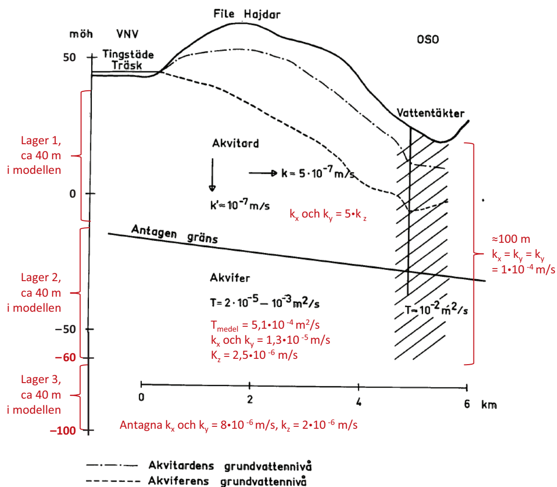
Figur 1. Generell profil över bergakviferen vid Slite–Filehajar.
