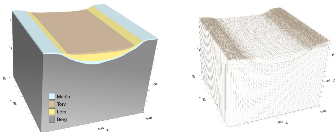
Figur 9. Numerisk modelluppställning för Typområde Lerslätt: konduktivitetslager (till vänster), och numerisk beräkningsgrid (till höger).
